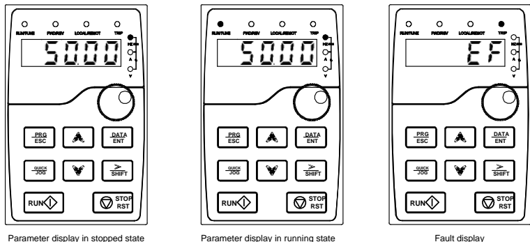
Рис. 5–2 Состояния дисплея
