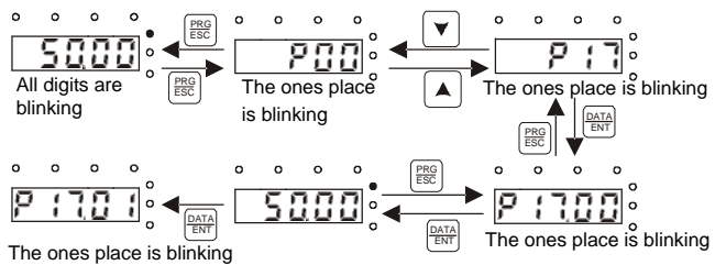
Рис. 5–5 Просмотр параметра
