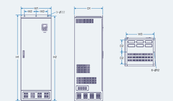
Напольный монтаж преобразователей 350—500кВт
