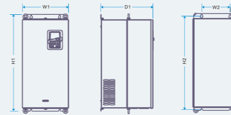
Фланцевый монтаж преобразователей 18 ~ 55кВт
