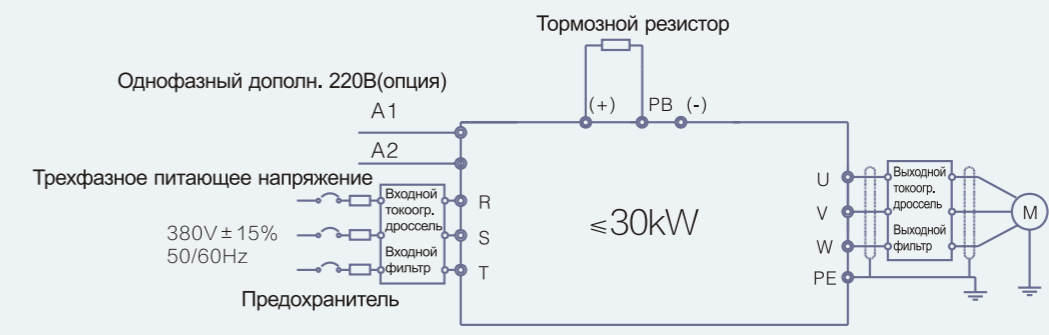
Схема подключения главной цепи
