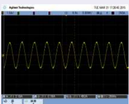
Форма тока при стабильной работе в режиме векторного управления на частоте 2000Гц
