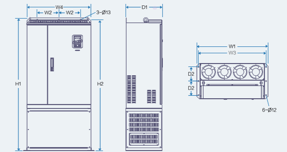
Напольный монтаж преобразователей 350—500кВт
